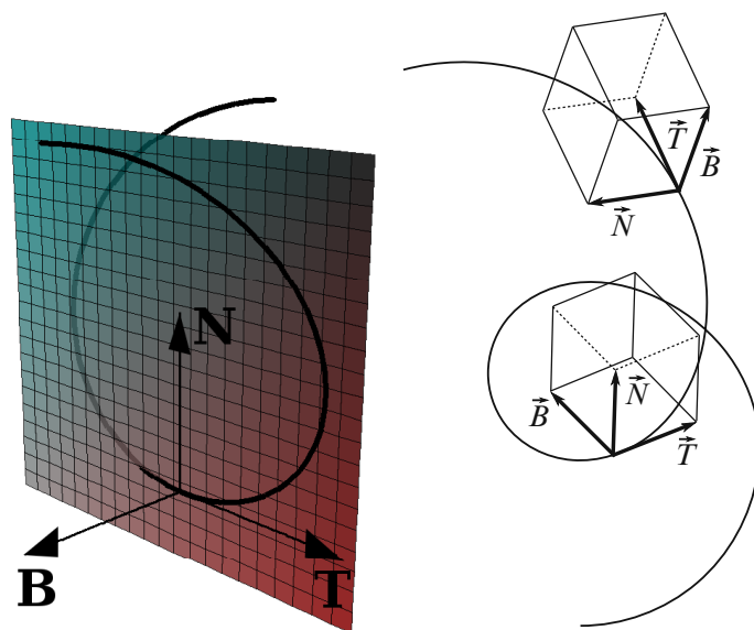
图 1.33: Frenet 标架
