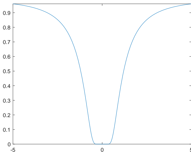
图 1.19: f(x) 的图像
