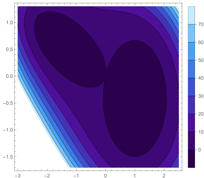
图 3.3: “8”字形水平集
