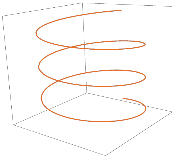
图 1.28: \mathbb{R}^3 中的螺线
